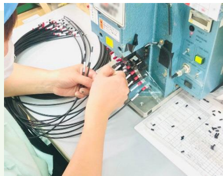
【ハーネスケーブル圧着加工作業（本社工場）】
